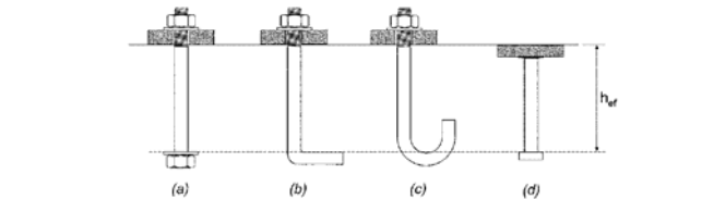
(A) 預埋式錨栓
