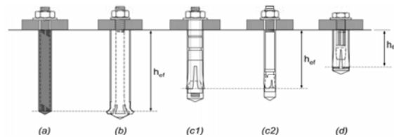
(B) 後置式錨栓
